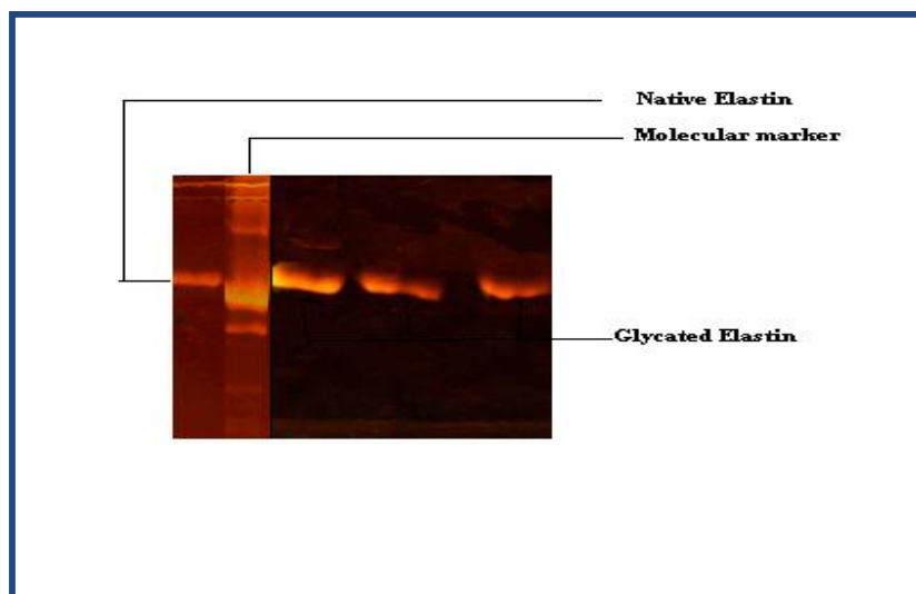
Fig3:- m-PAGE –electrogram .
